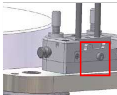
Abb.16 b: Einstellung des Neigungswinkels
