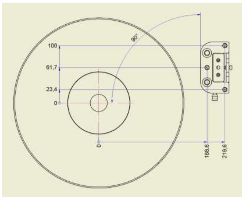
Abb.4: Bohrschablone
